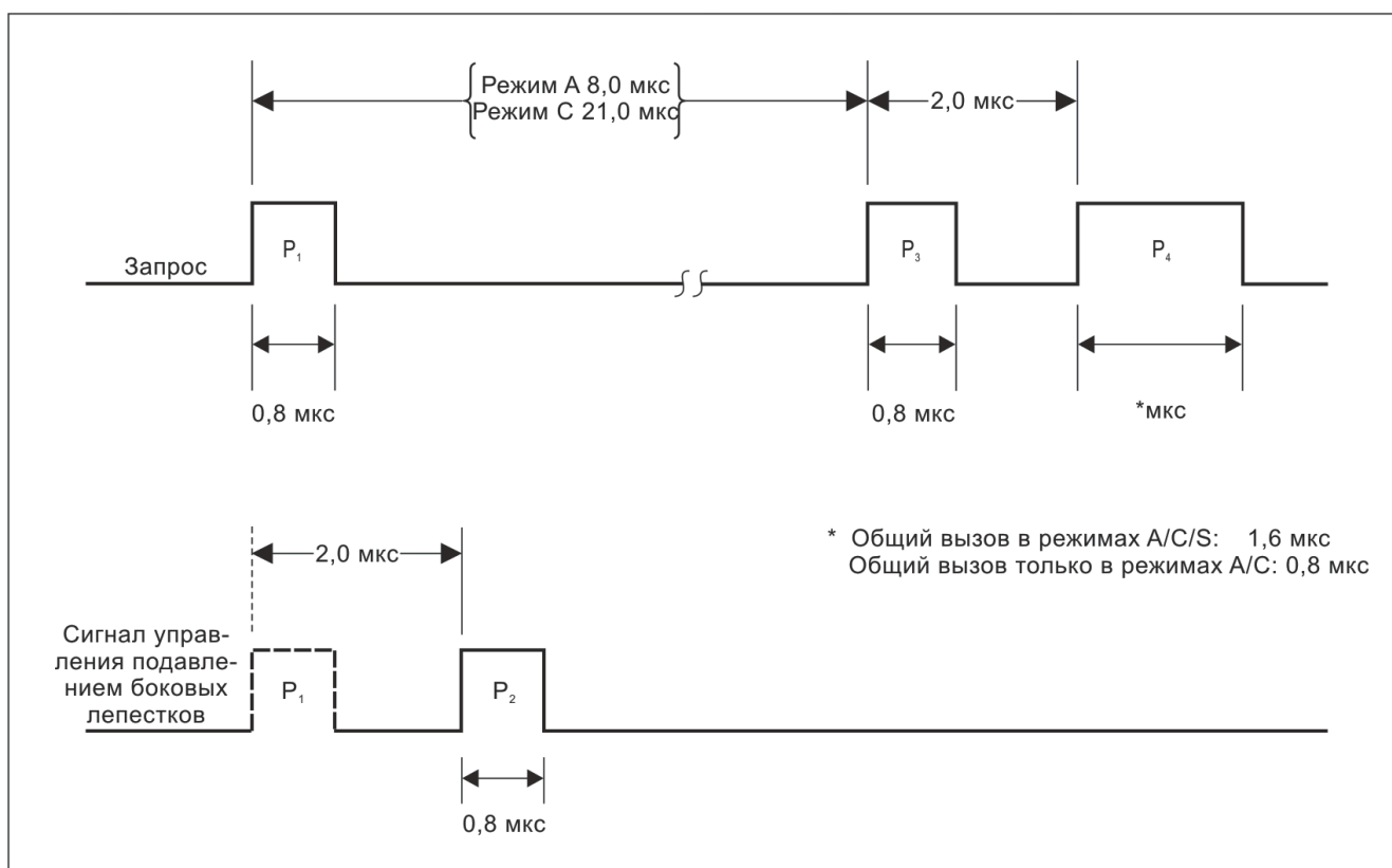
Рис. 2. Последовательность импульсов межрежимного запроса
