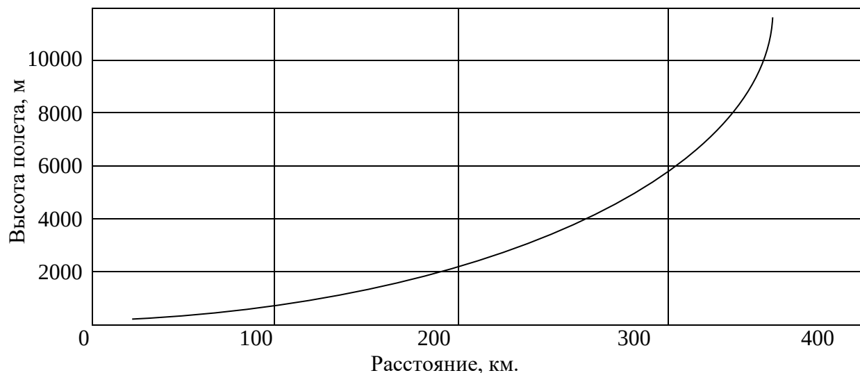
График дальности двусторонней радиосвязи с воздушными судами
