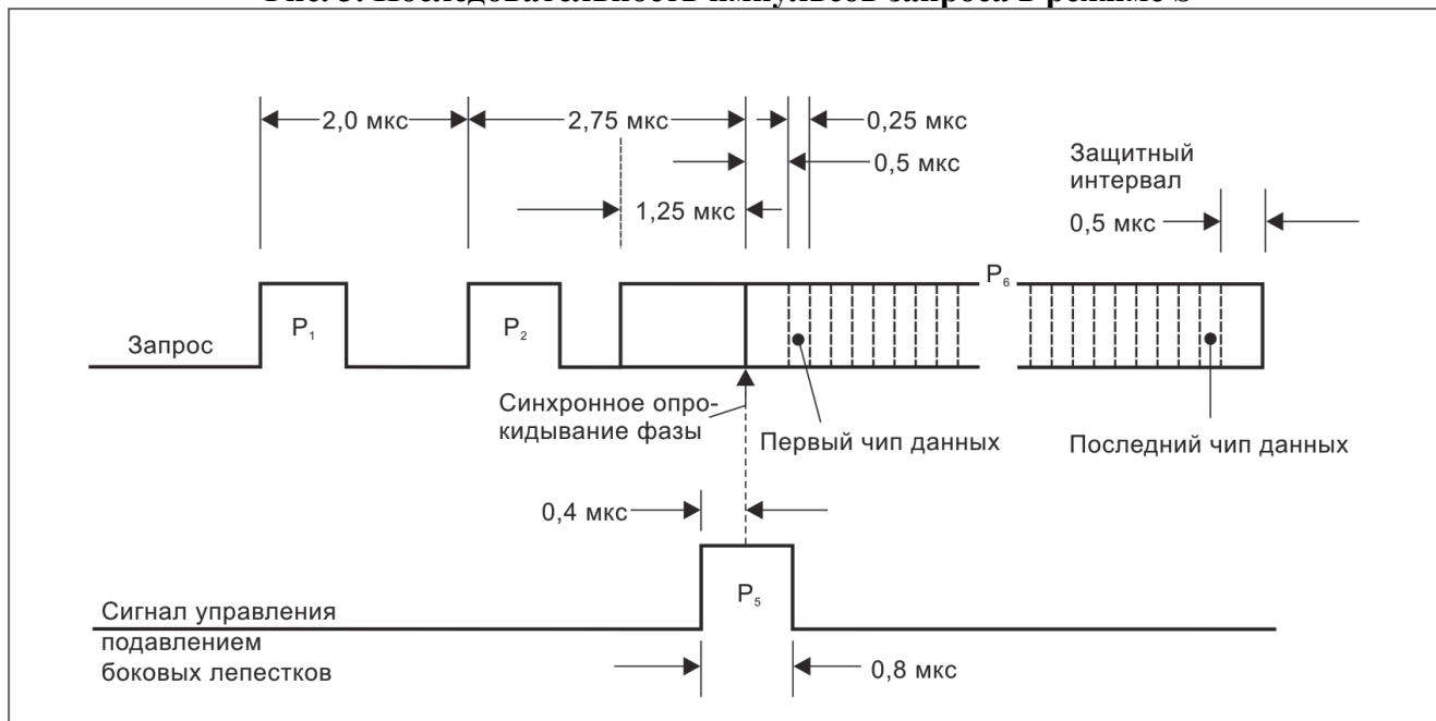
Рис. 3. Последовательность импульсов запроса в режиме S
