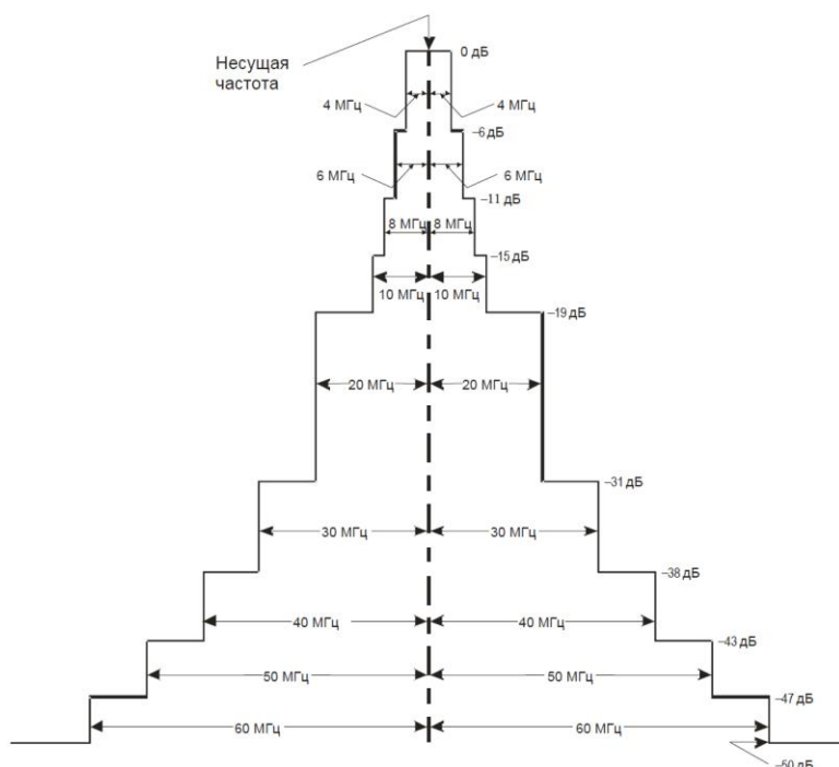
Рис. 1. Требуемые предельные значения спектра для передатчика запросчика
