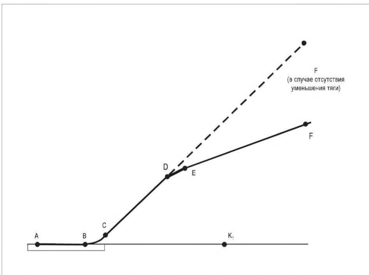
Рис. А2-5. Исходные характеристики профиля полета самолета
