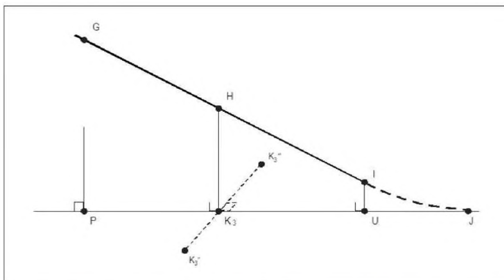
Рис. А2-9. Характеристики исходного профиля захода на посадку вертолета
