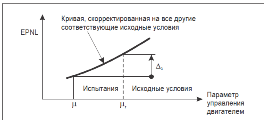
Рис. A2-12. Поправка на шум источника
