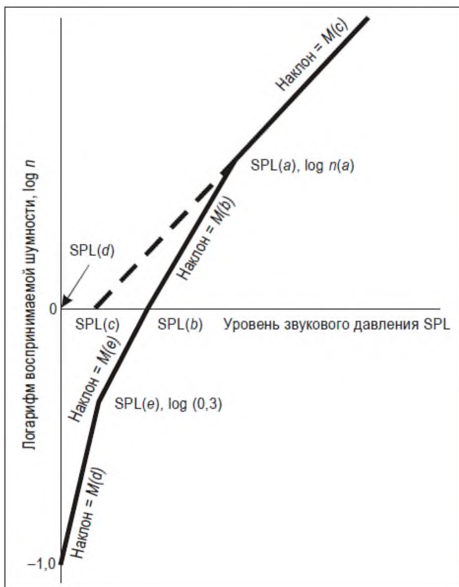
Рис. А2-3. Зависимость воспринимаемой шумности от уровня звукового давления
