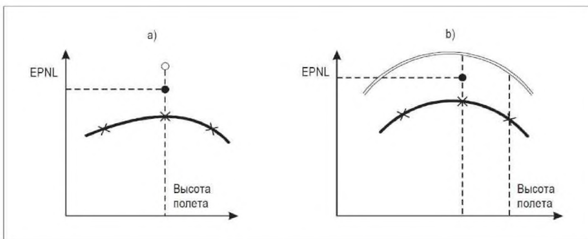
Рис. А2-13. Поправки на боковую асимметрию
