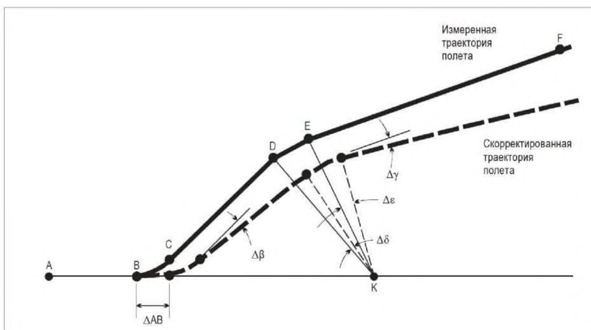
Рис. А1-5. Сравнение измеренного и скорректированного профилей взлета
