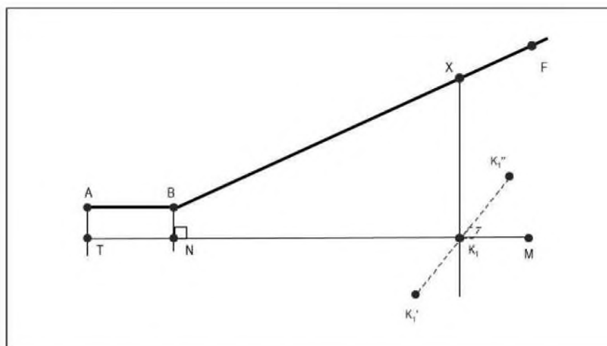
Рис. А2-7. Характеристики исходного профиля взлета вертолета
