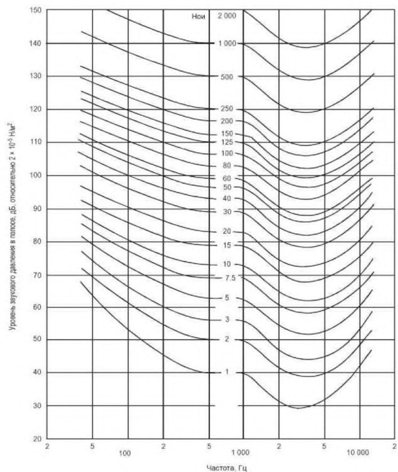
Рис. А5-1. Кривые воспринимаемой шумности
