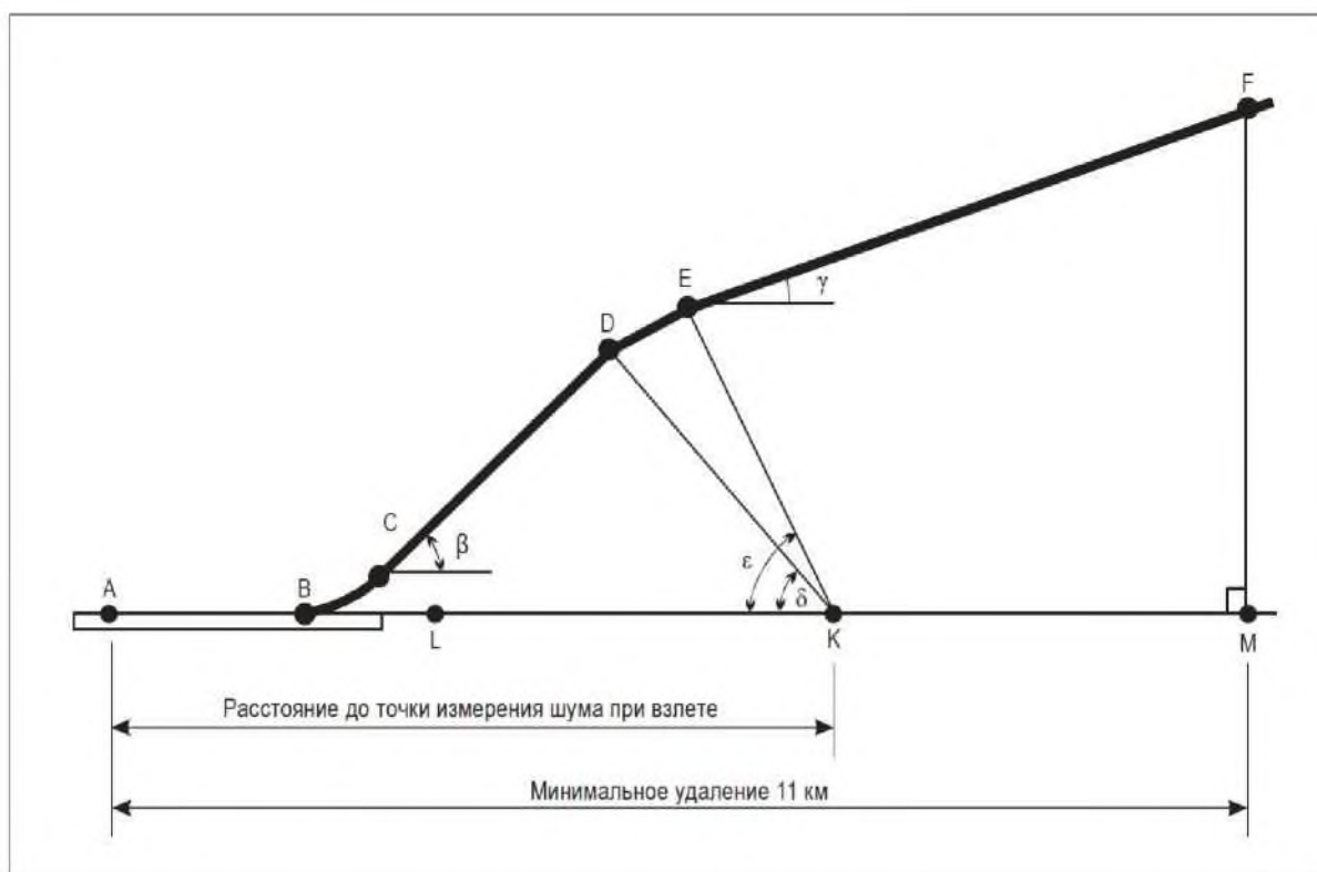
Рис. А1-4. Измеренный профиль взлета
