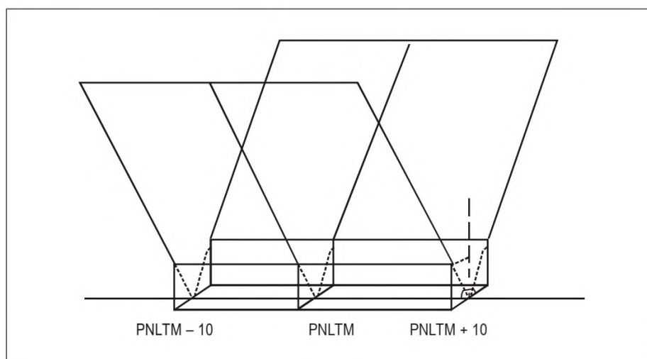
Рис. 8-1. Допуски на боковое отклонение вертолета
